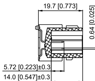
SEC:A-A
