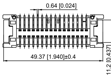
SEC:A-A
