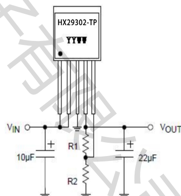
HX29302-TP典型应用
