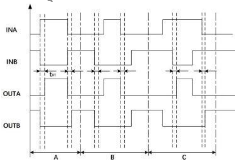
图 36 各情况下死区时间时序图
