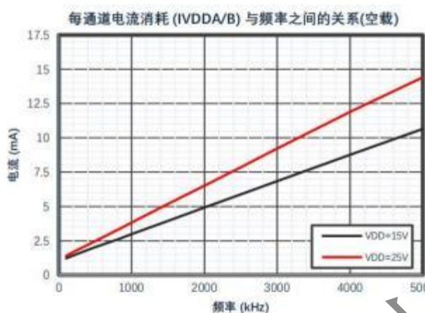
图 3 电流消耗(IVDDA/B)与频率间的关系(空载)
