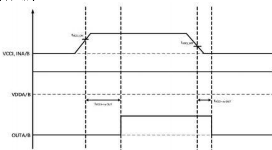
图 30 VCCI UVLO 触发/恢复到输出响应的延迟时间
