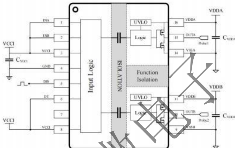
图 26 使能响应时间的测试电路
