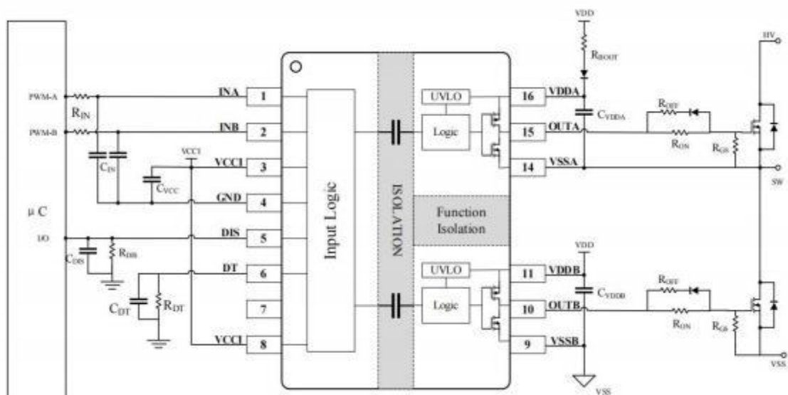
图 1 典型应用图
