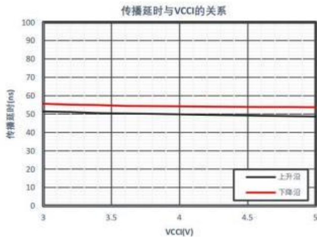
图 7 传播延时与 VCCI 的关系
