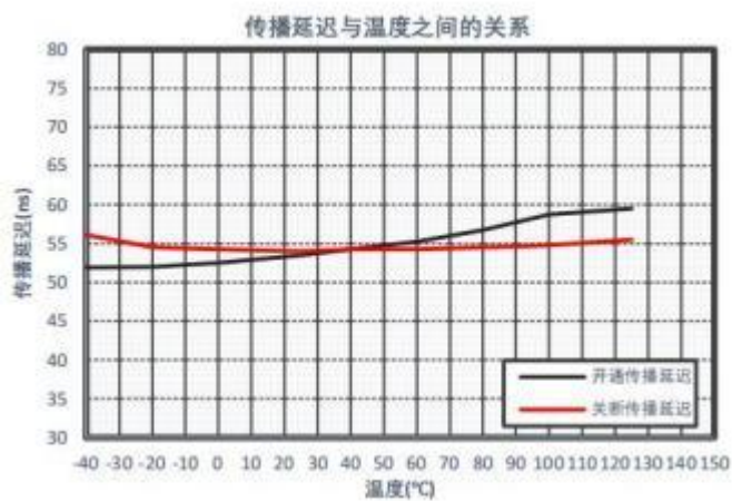
图 12 传播延迟与温度之间的关系
