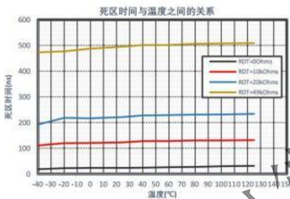
图 21 死区时间与温度间的关系
