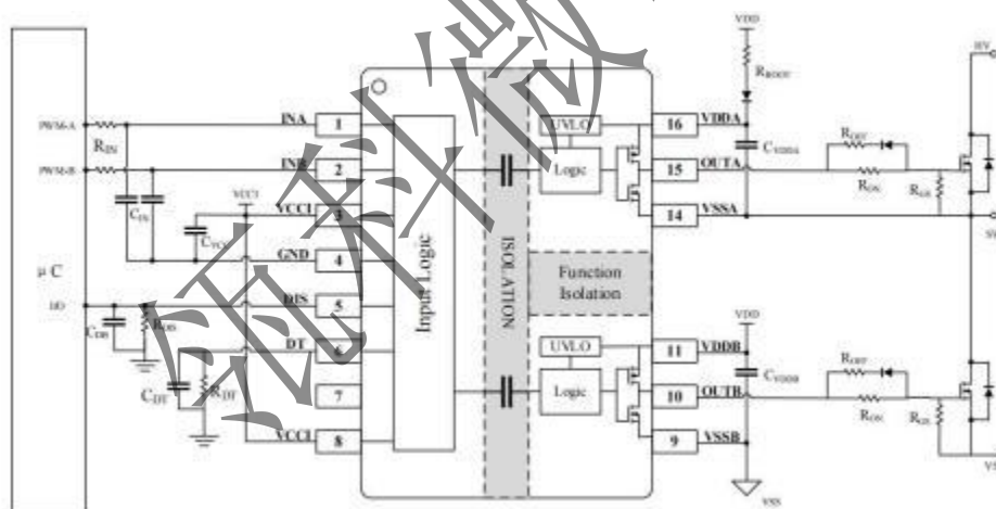
图 37 典型应用参考方案原理图
