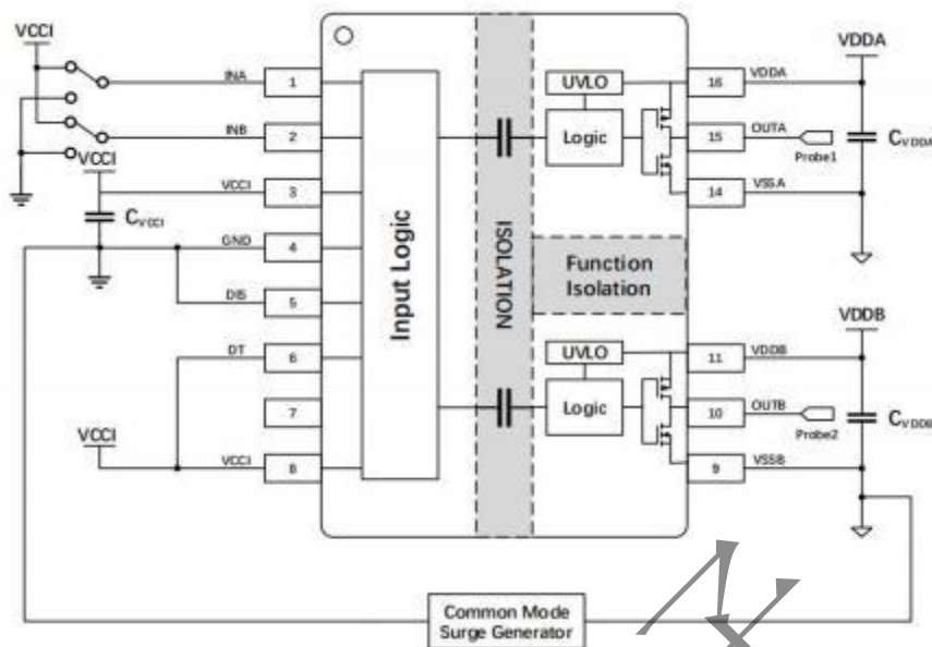
图 32 CMTI 测试电路
