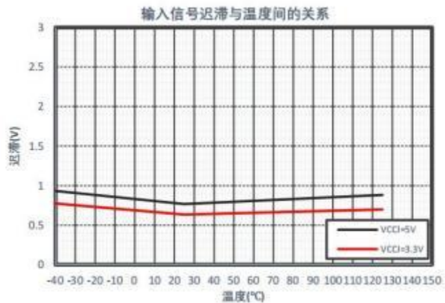
图 19 输入信号迟滞与温度间的关系
