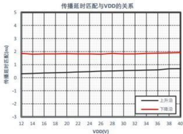
图 8 传播延时匹配与 VDD 间的关系
