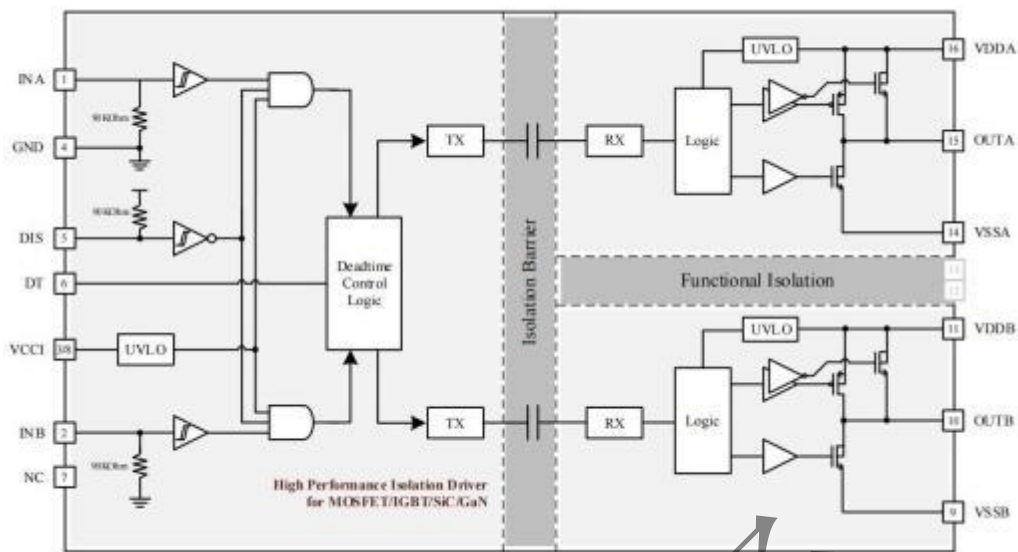
图 33 功能框图
