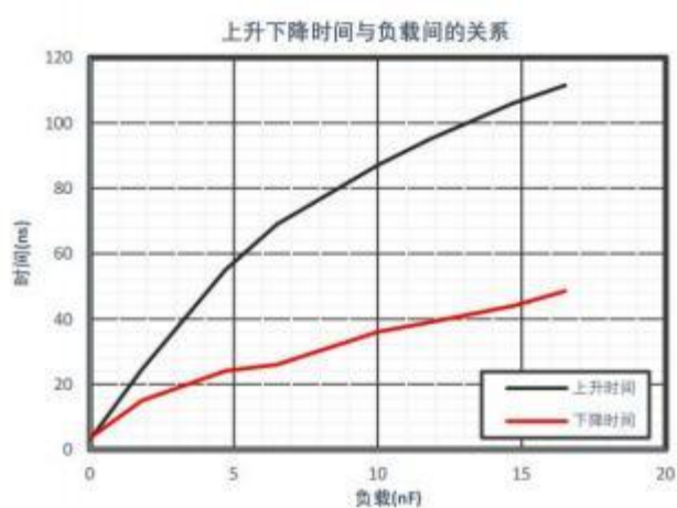
图 6 上升下降时间与负载间的关系
