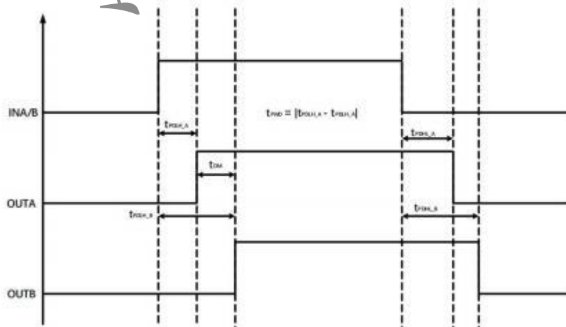
图 25 传播延时、脉宽失真与传播延迟匹配的时序图
