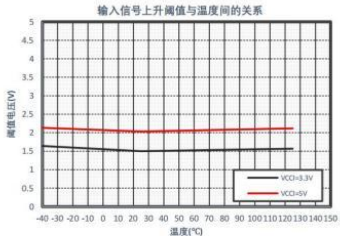
图 20 输入信号上升阈值与温度间的关系
