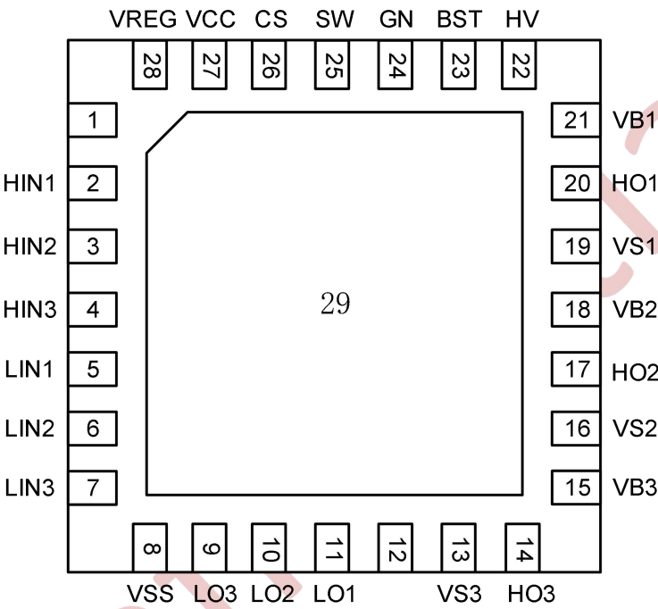
图 7-1 QFN28 顶视图
