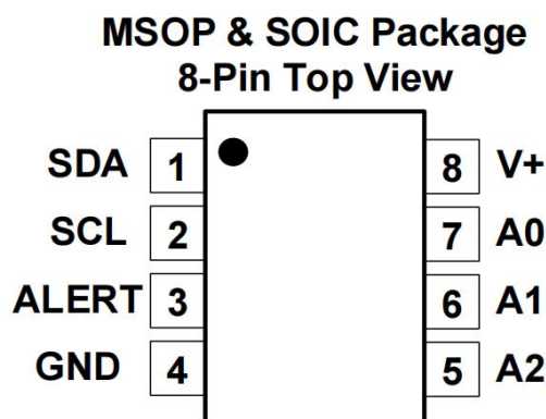
引脚功能
