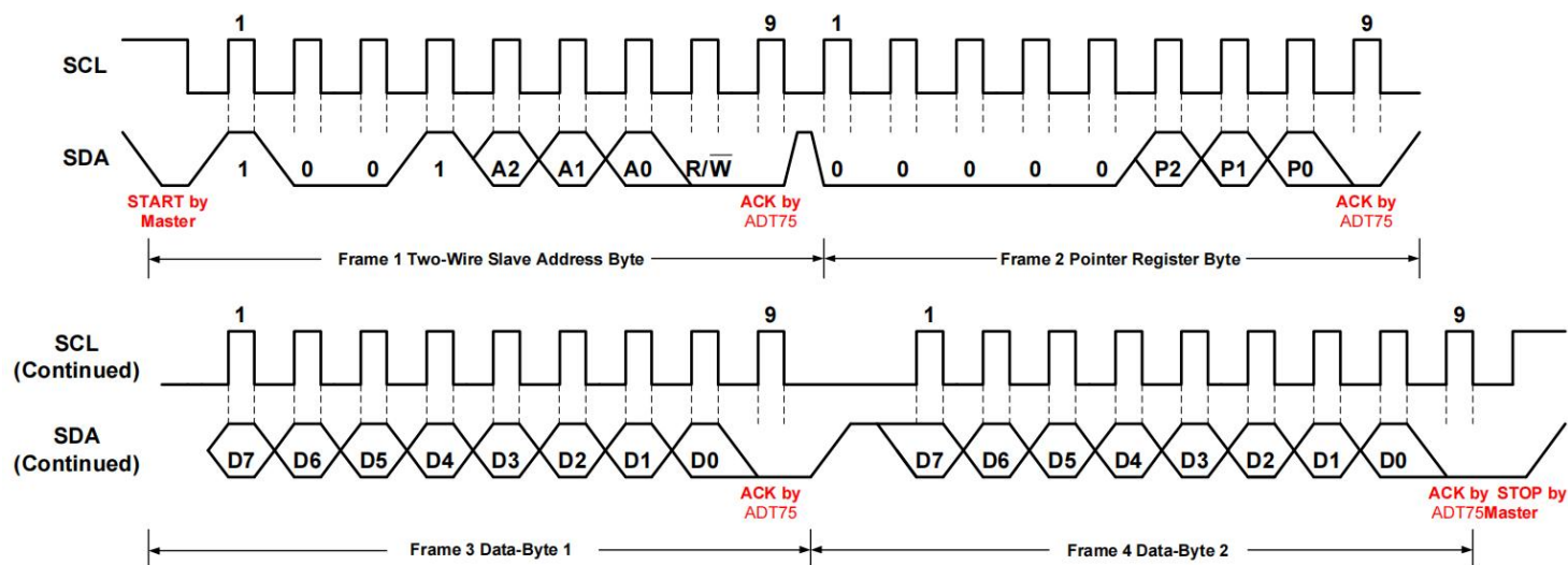
图 3 两线制写命令时序图
