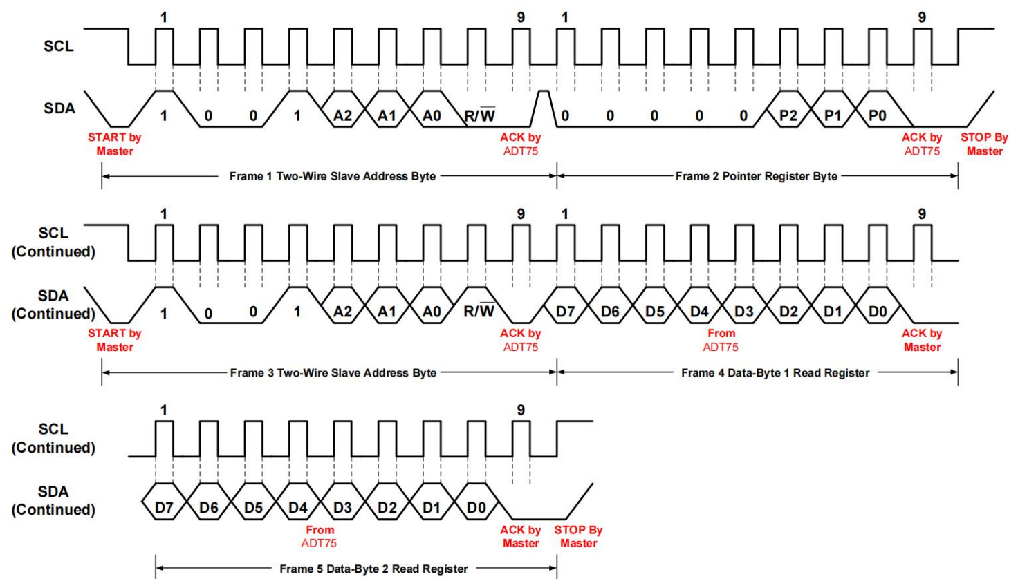
图 4 两线制读命令时序图
