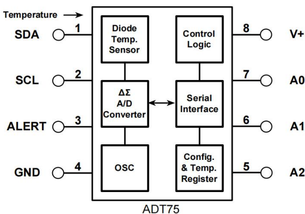
图 1 ADT75内部各模块示意图
