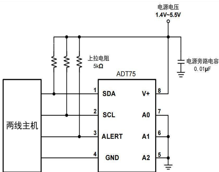
图 7 ADT75的典型连接方式
