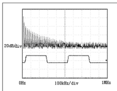
图11：传输20kHz信号时 SP3485EN+TD驱动器 输出波形和FFT图
