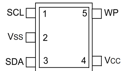
SOT-23
