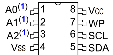
SOIC/TSSOP (Top view)
