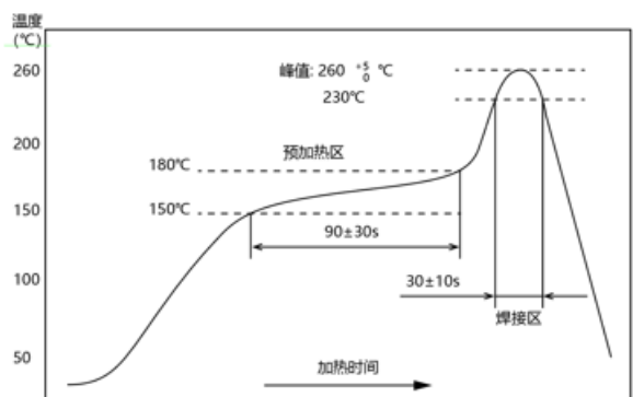
回流焊曲线图
