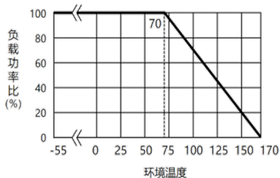
功率曲线
