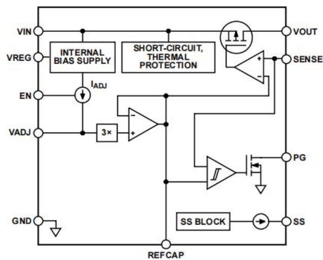
图 3 功能框图
