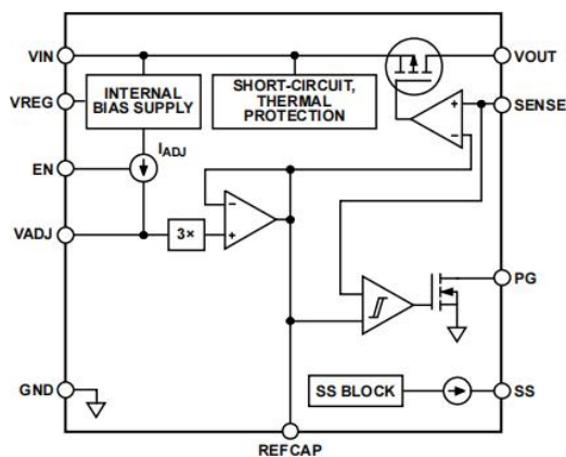
图 4 功能结构框图
