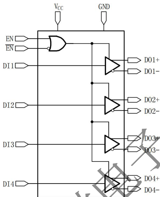
图9 功能框图
