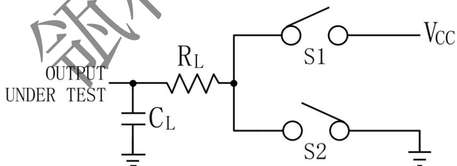
图 6 启用/禁用延迟测试电路图
