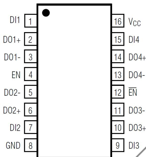
图 2 引脚排列图（顶视图）
