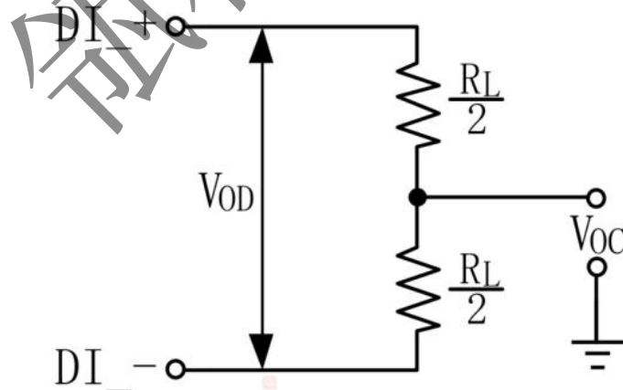
图 3 差分测试电路图
