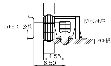
组装示意图
