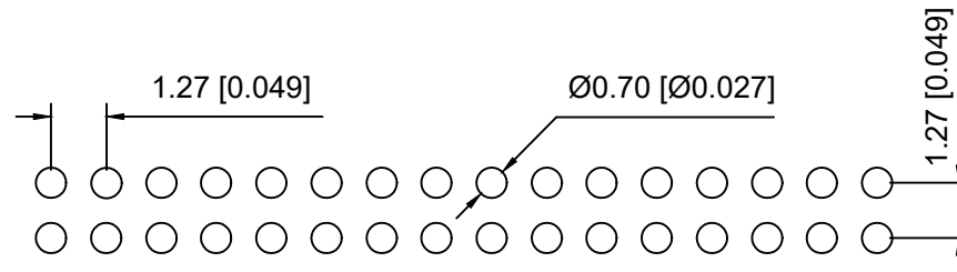
P.C.B LAYOUT
