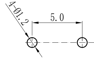
PCB线路板安装图(±0.1)
