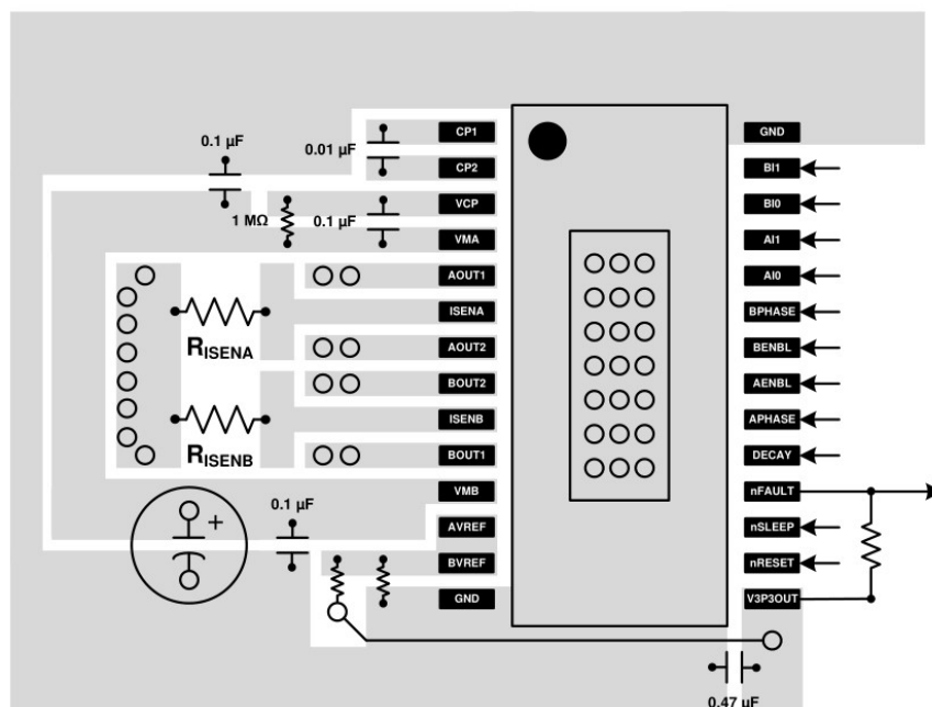
图 9. SS8812T 布局实例
