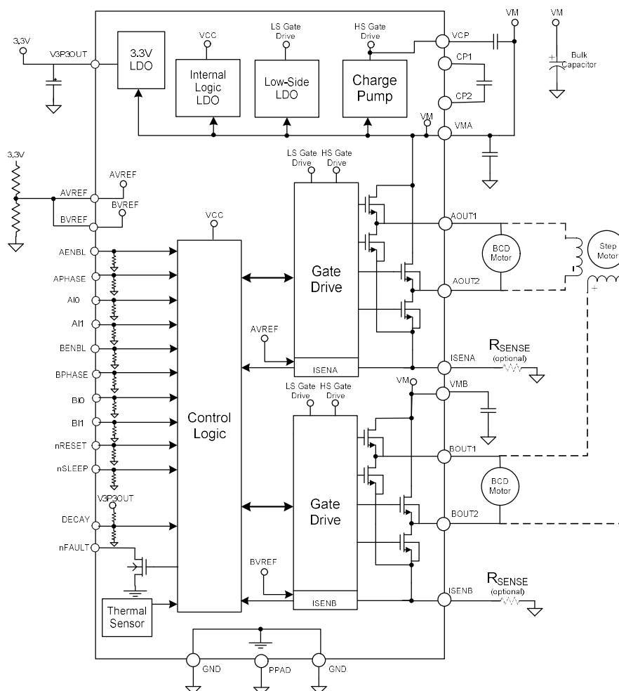
图 3. 功能结构框图
