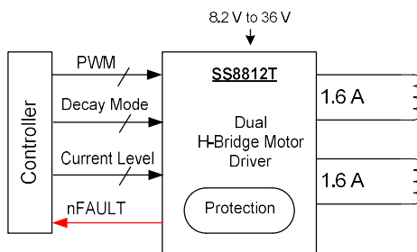
图 1. 典型应用原理图
