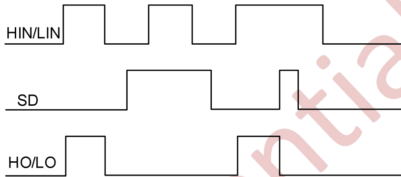
图 8-1 NSG2113 输入输出时序波形
