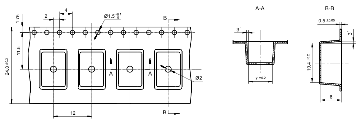
载带外形图 (S1型: 短脚表面贴装型)
