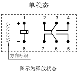
接线图 (底视图)
