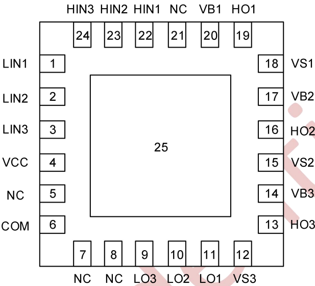
图 7-1 G2063Q QFN24 顶视图
