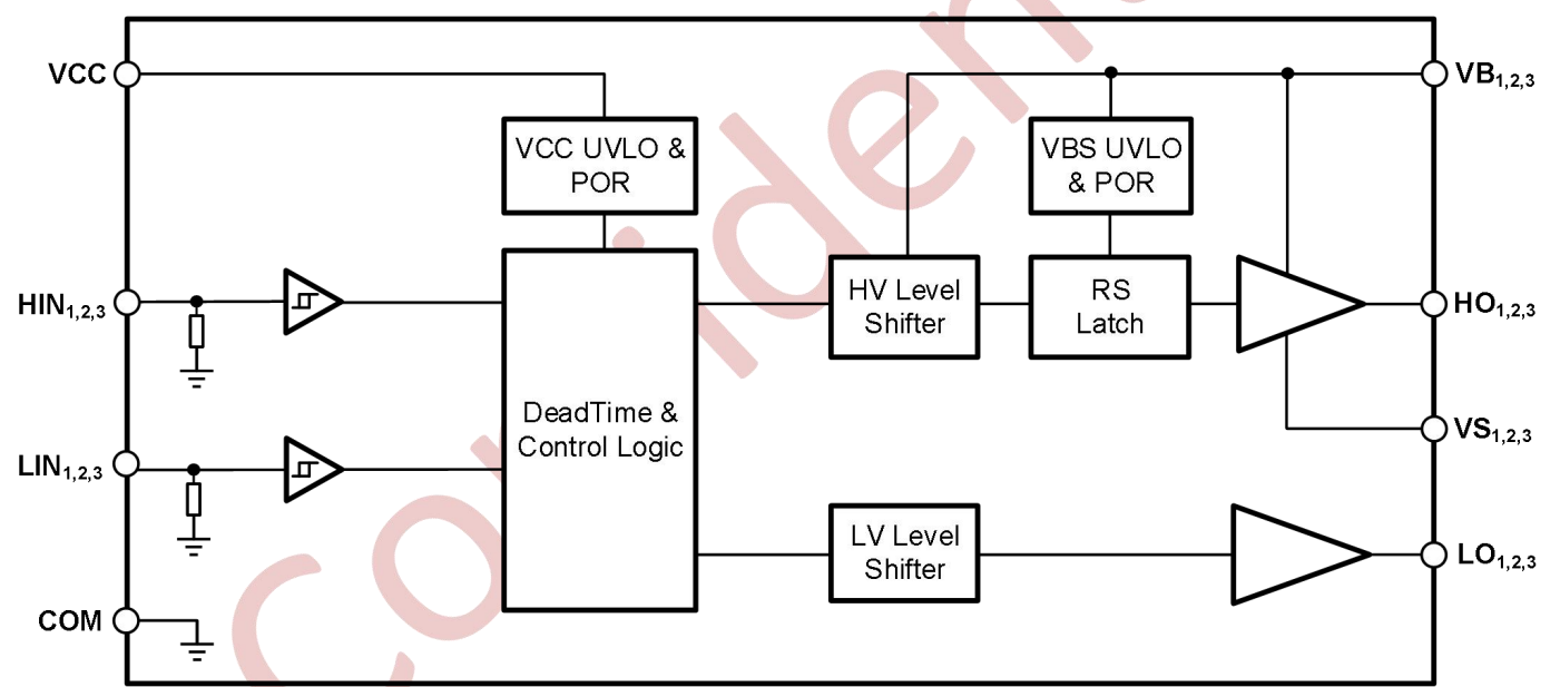
图 10-1 G2063Q 功能框图
