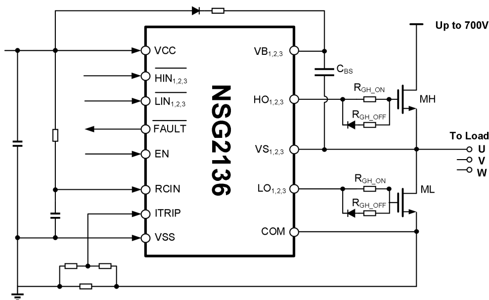
图 10-7 典型应用电路图
