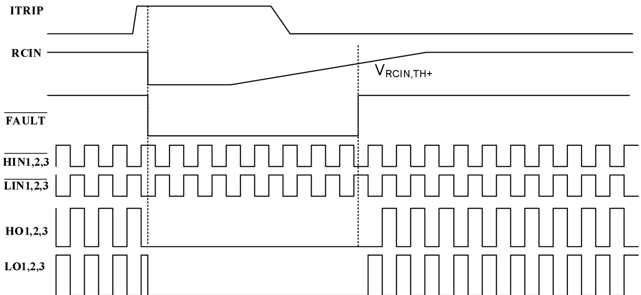
图 10-5 过流保护波形定义
