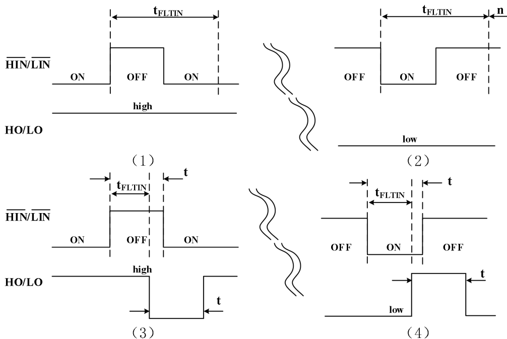
图 10-2 输入滤波波形定义
