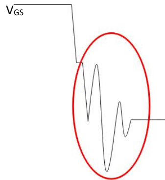
图 10-10 栅极振铃现象
