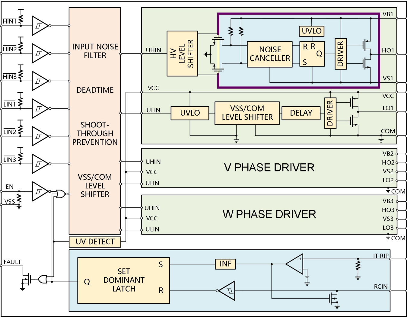
图 10-1 NSG2136 功能框图
