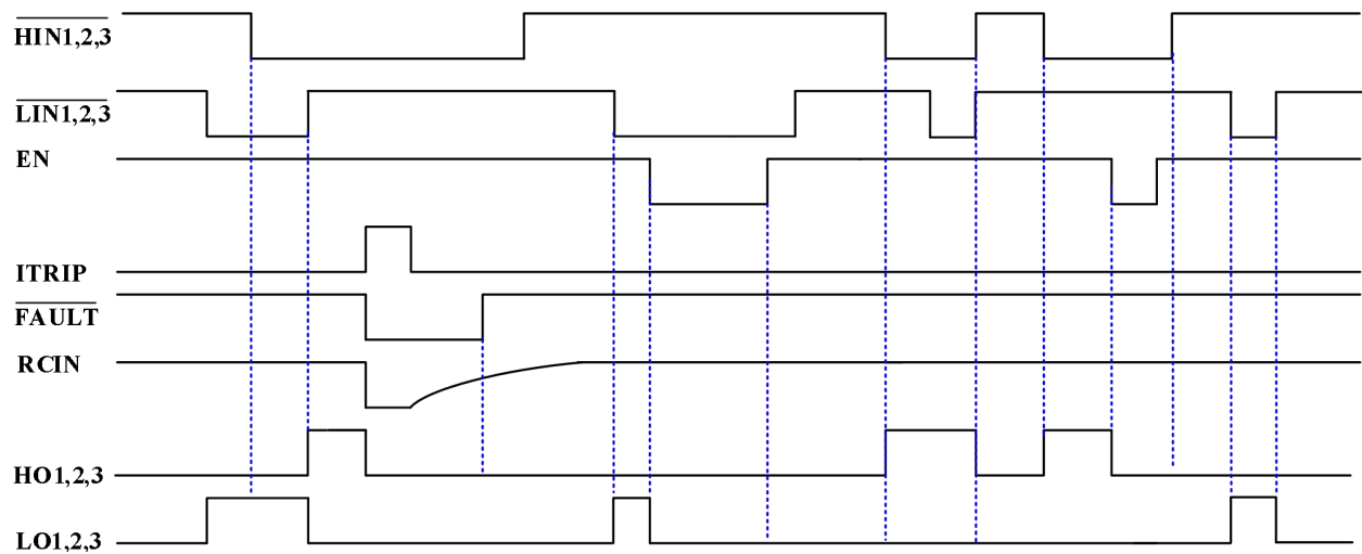
图 9-1 输入输出时序波形
