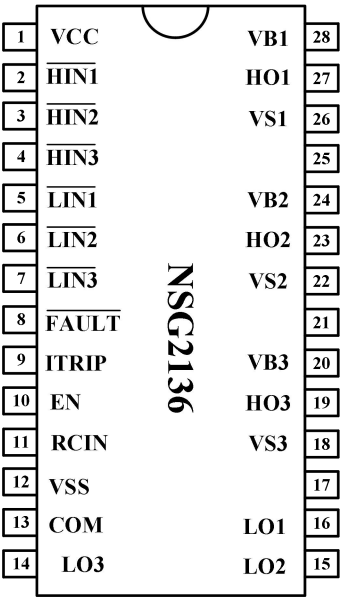
图 7-1 28-脚 SOP 顶视图
