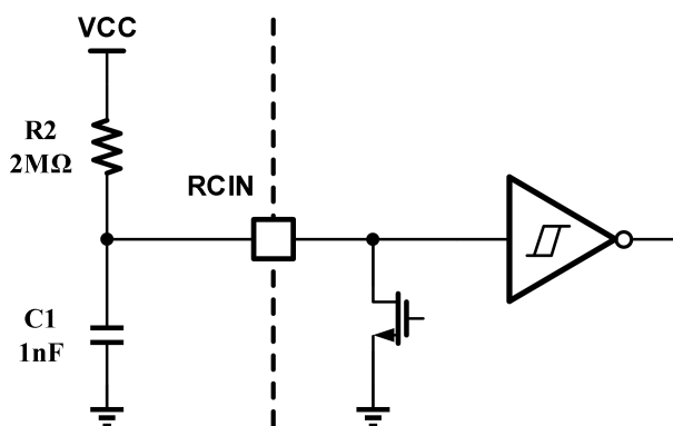
图 10-6 RCIN 引脚框图
