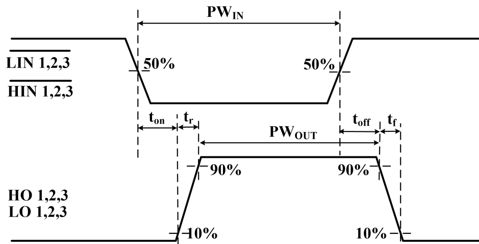
图 9-2 传输时间波形定义
