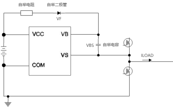
图 10-8 自举电路基本结构
