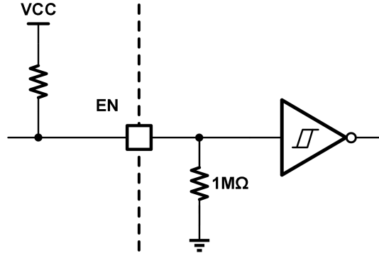
图 10-4 EN 引脚框图
