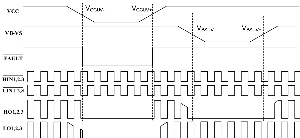
图 10-3 欠压功能波形定义
