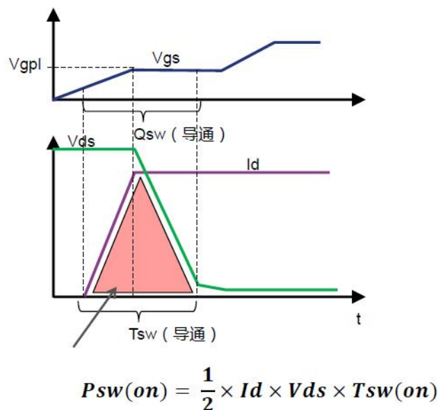
图 10-9 阻性负载条件下的 MOS 开关损耗
