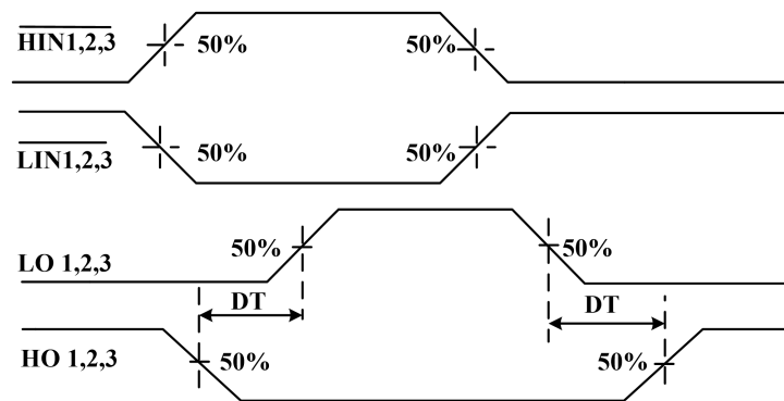
图 9-4 开关时间波形定义
