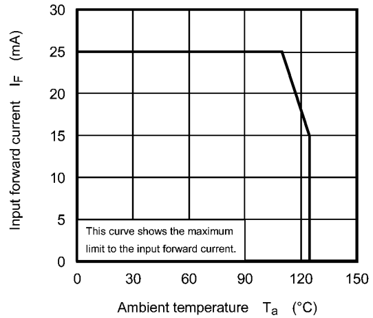
Fig. 13.2.2 I_F - T_a
