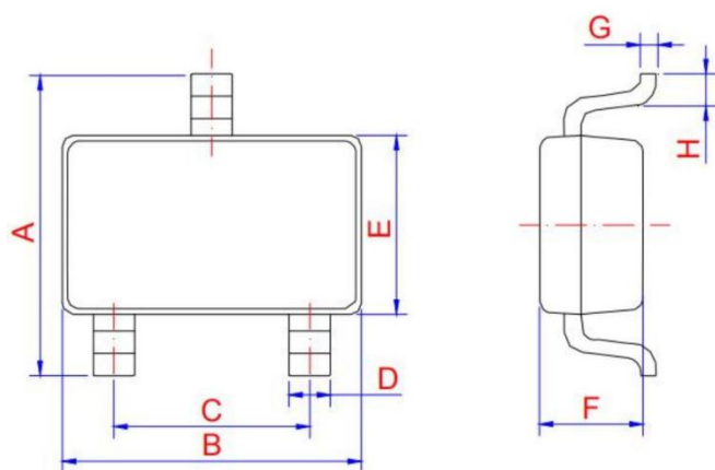
SOT-23-3L
