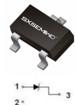
SOT-23
