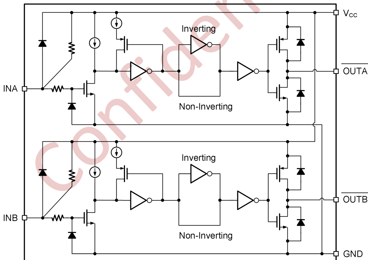
图 10-1 NSG4426 功能框图
