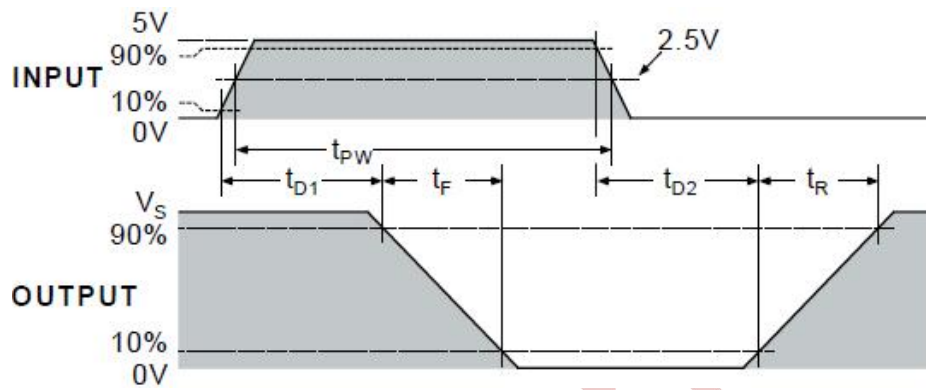
图 9-1 输入输出(反相)波形图
