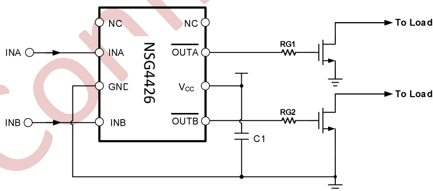
图 11-1 NSG4426 反相典型应用电路图
