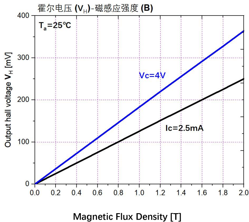
图 4. 霍尔电压-磁感应强度
