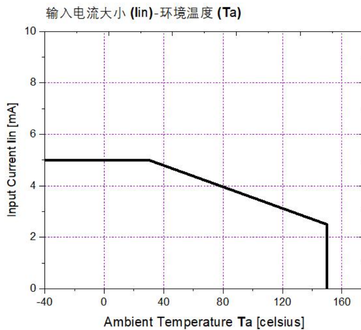
图1. 最大输入电流-环境温度
