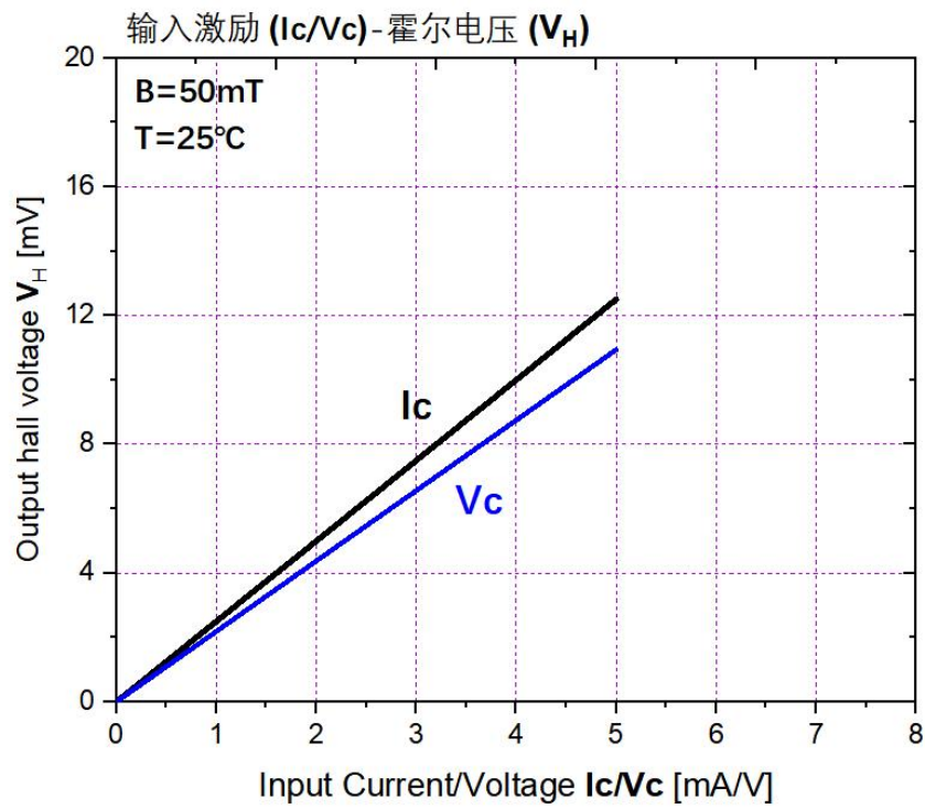
图 6. 输入电流/电压-霍尔电压
