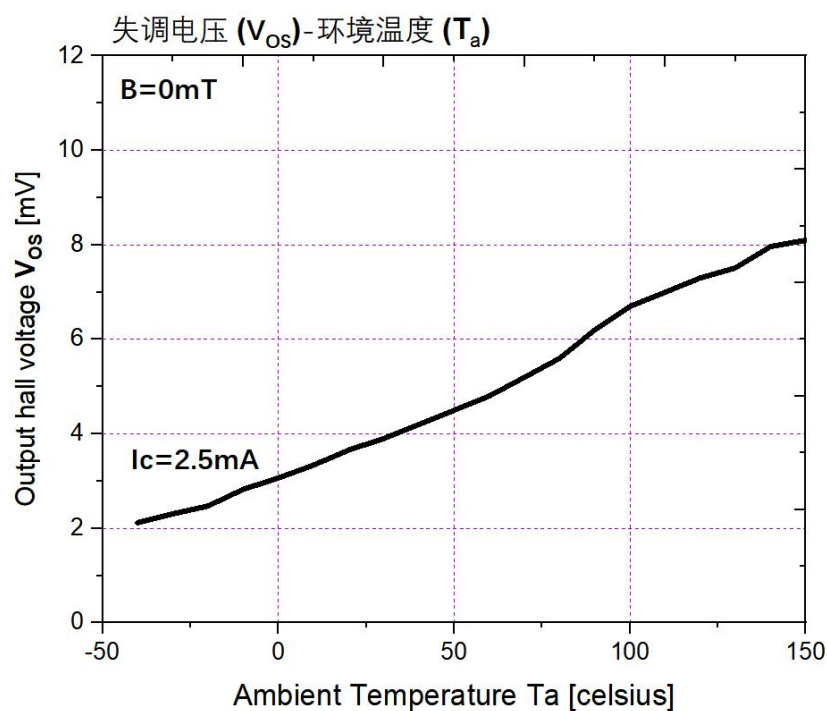
图 5. 失调电压-环境温度
