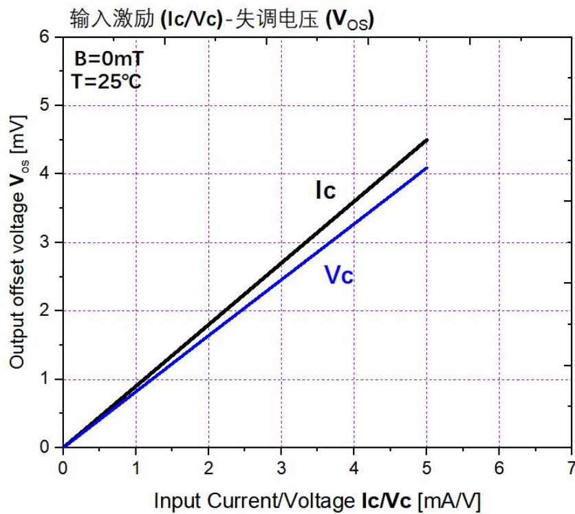
图 7. 输入电流/电压-失调电压
