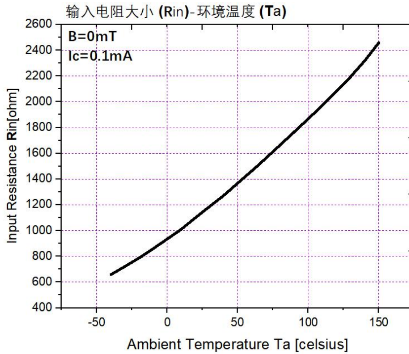
图 2. 输入电阻-环境温度
