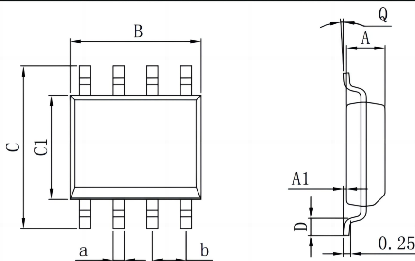
SOP8
