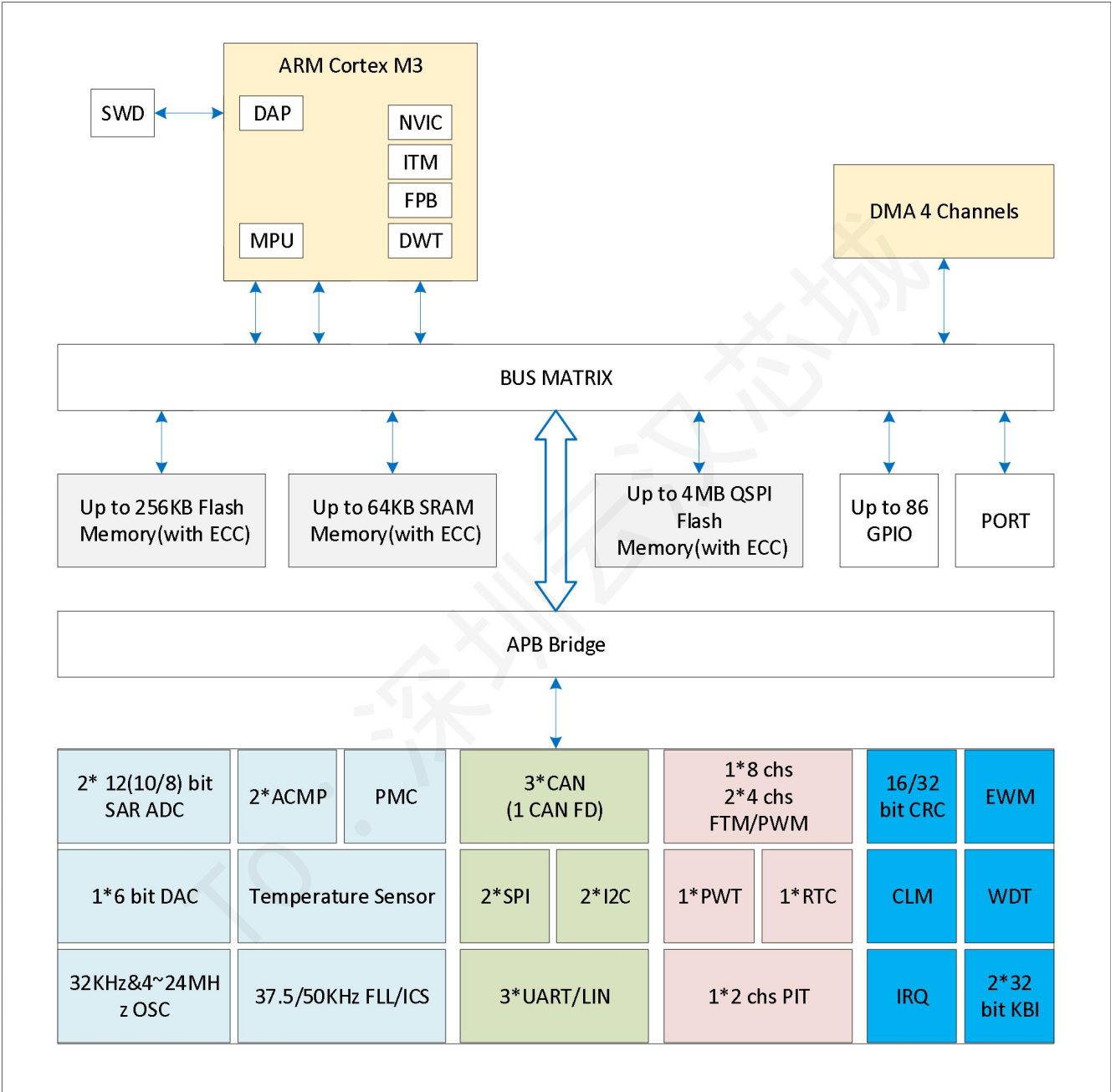
图 2-1 芯片结构图
