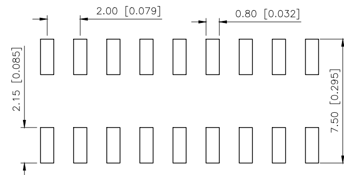
P.C.B. LAYOUT
