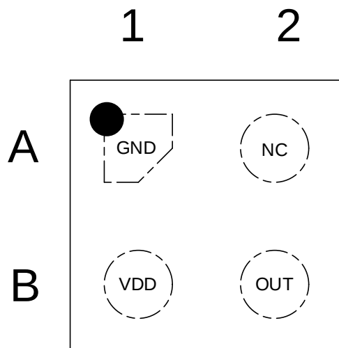
AW86511EBCFDR (Top View)
