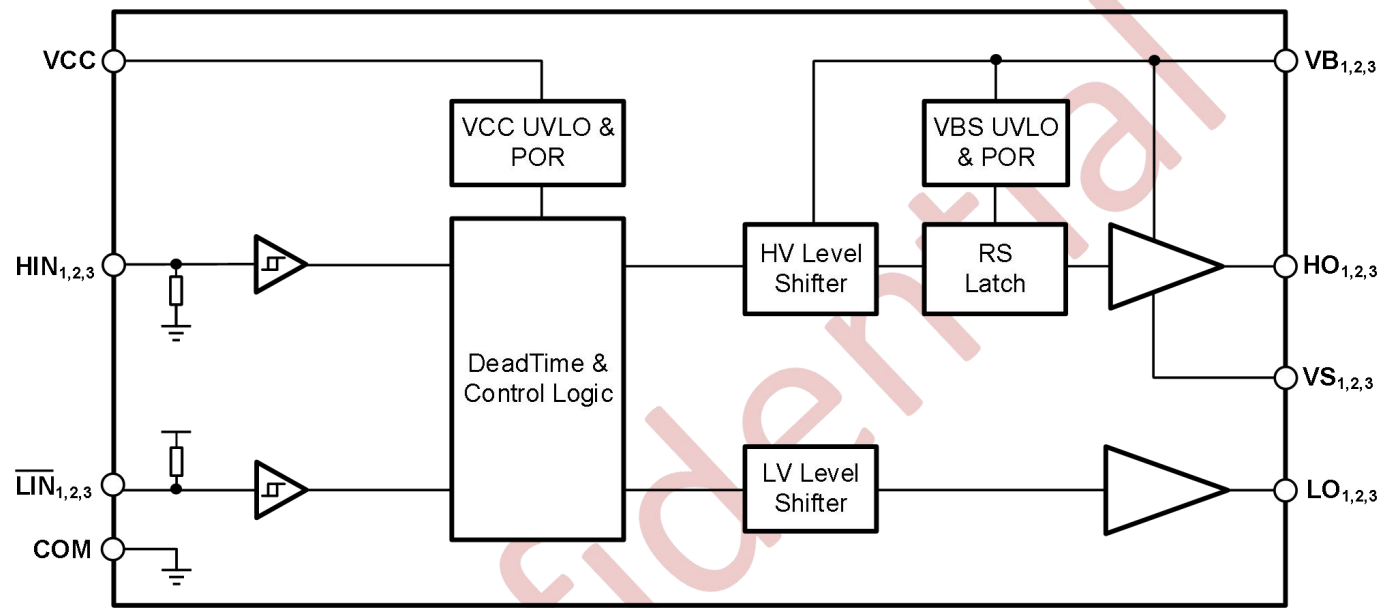
图 10-1 G2060 功能框图
