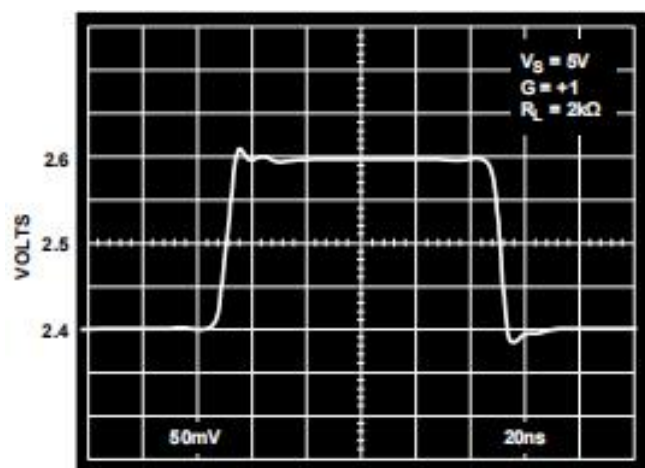
图 7 200mV 输入，输出过冲实测图
