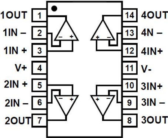
图 2 引脚排列图（顶视图）
