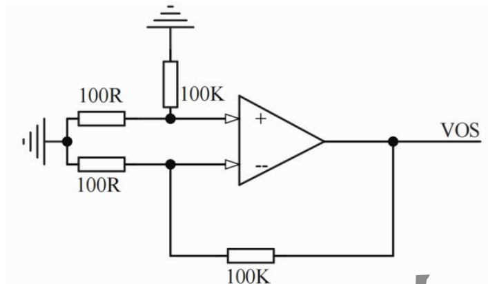
图 4 输入失调电压测试电路
