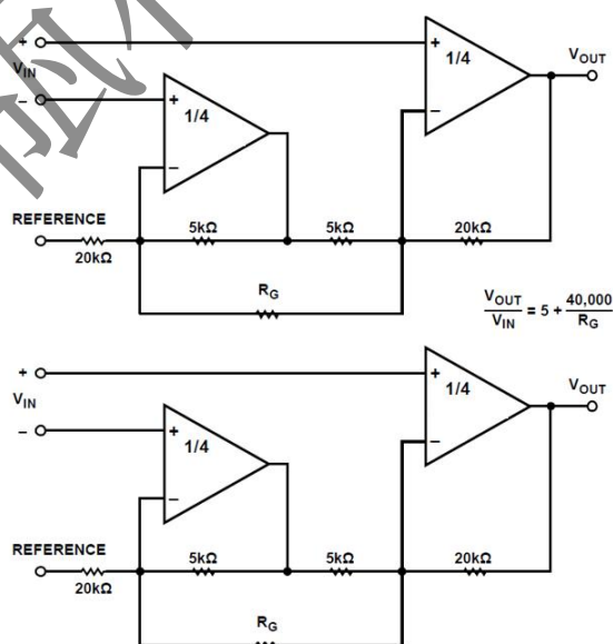
图 8 双路低功率运算放大器电路
