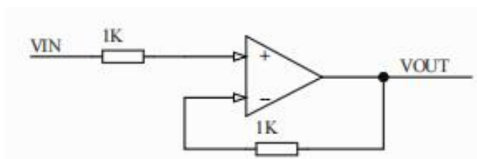
图 6 过冲测试电路
