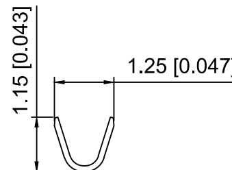
SEC:B-B
