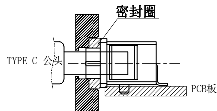
组装示意图
