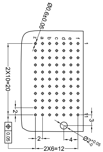
固定PCB 板尺寸 (公差 ± 0.05)
