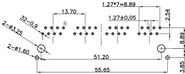
PCB参考图
