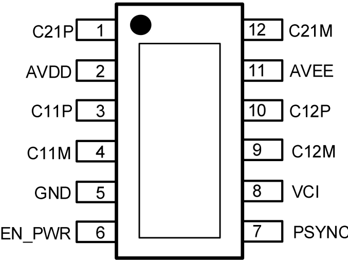
图 6-1 12-脚 TDFN 顶视图
