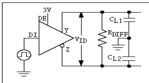
图 4:驱动器定时测试负载
