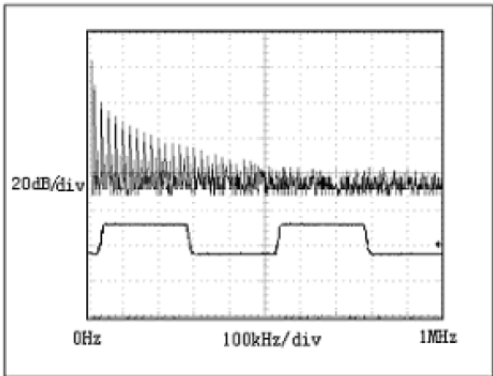
图11：传输20kHz信号时 MAX3485ECSA-TD驱动器输出波形和FFT图
