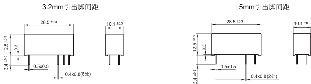
外形图
