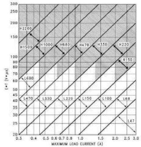
LM2576HV-ADJ
