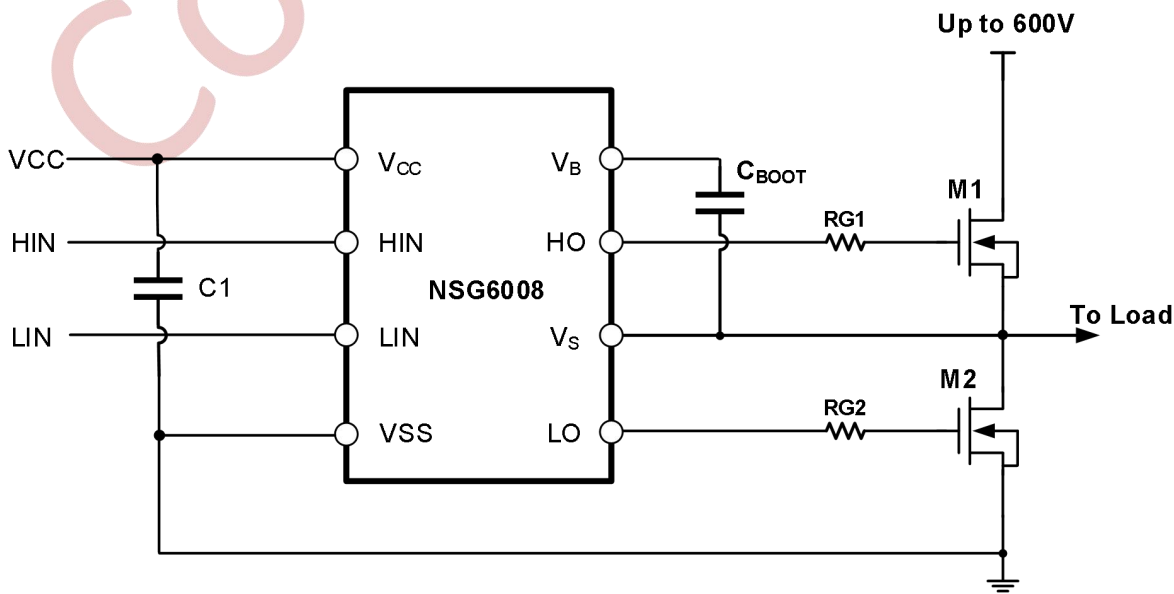
图 10-2 NSG6008 典型应用电路图
