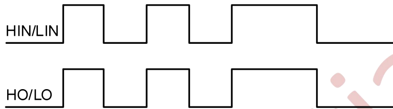
图 9-1 NSG6008 输入输出时序波形
