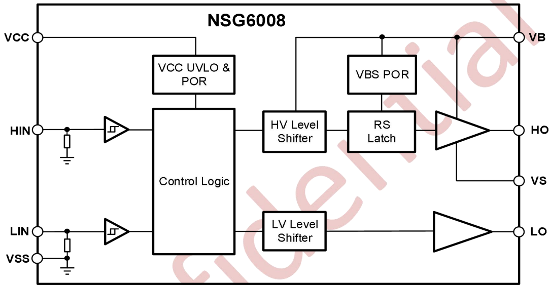
图 10-1 NSG6008 的功能框图
