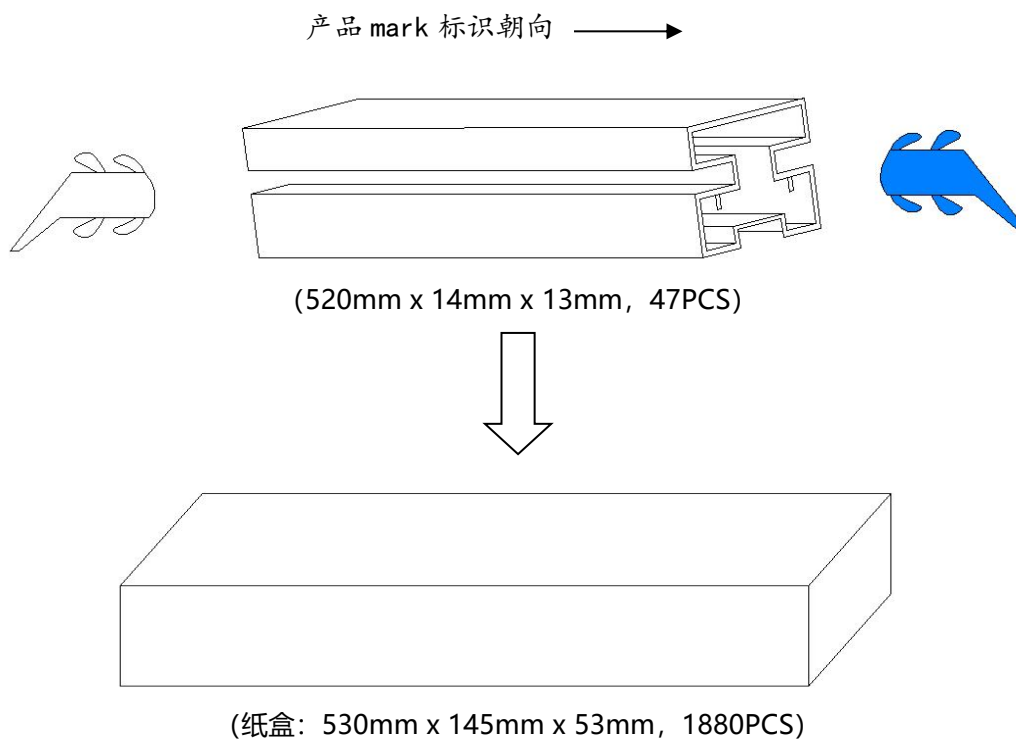
图 10.包装示意图
