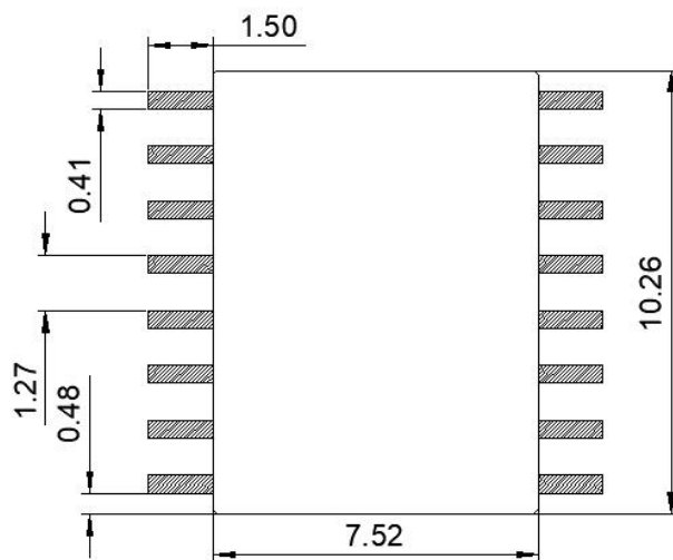
图 8. 推荐焊盘尺寸
