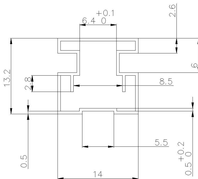
图 9.料管截面示意图
