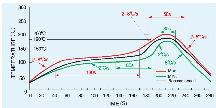
图 9.回流焊接
